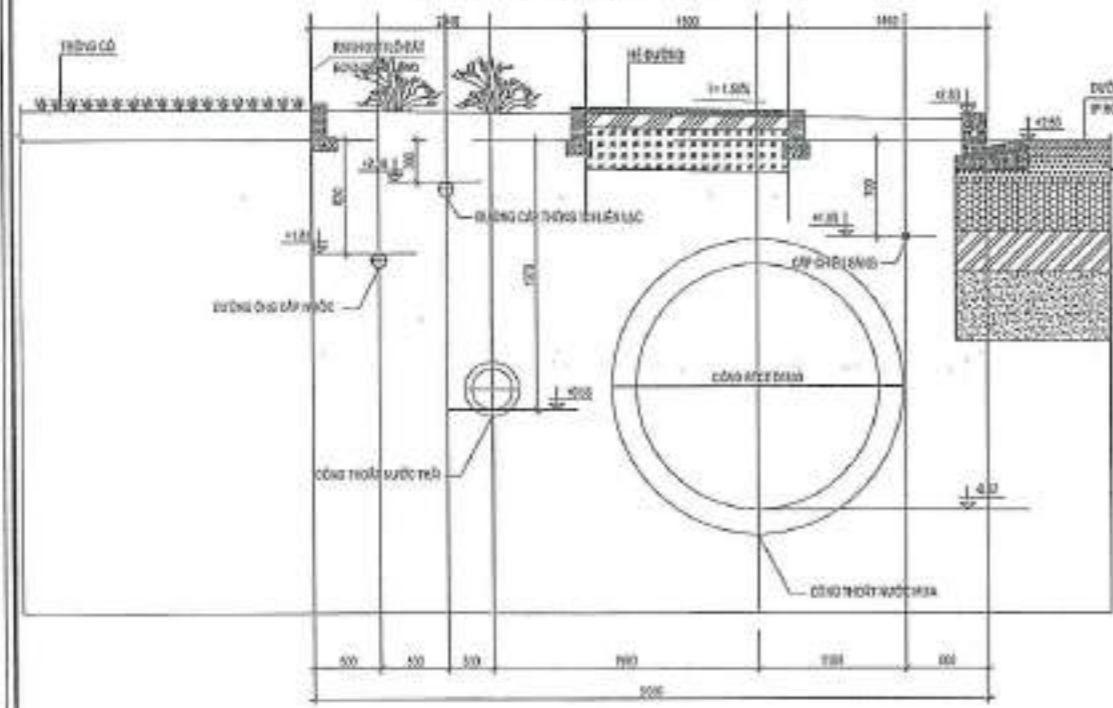
MẶT CẮT 2-2 (HIỆN TRẠNG) SECTION 2-2 (EXIST)
