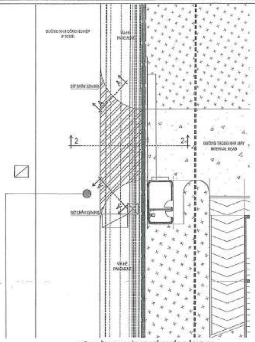
MẶT BẰNG ĐƯỜNG KẾT NỐI CÔNG 01 GATE 02 ROAD CONNECT PLAN
