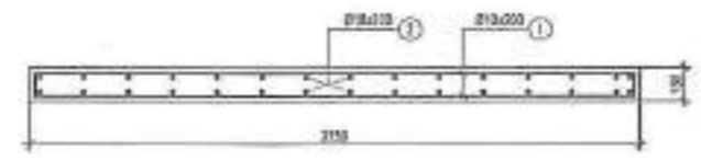
CHI TIẾT TẤM D.150 DETAIL PLATE T02
