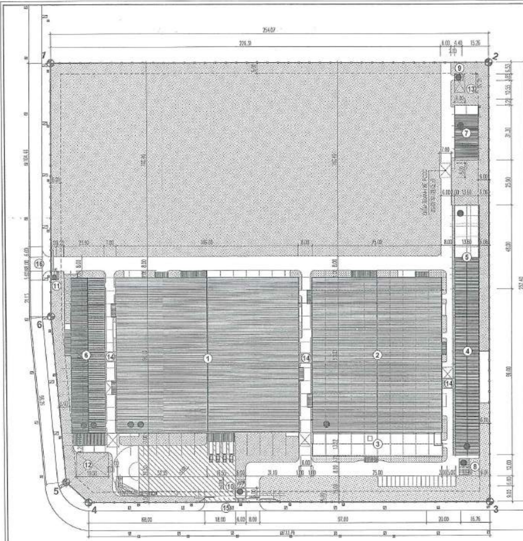
MẶT BẰNG TỔNG THỂ/总平面图 SCALE 1:500
