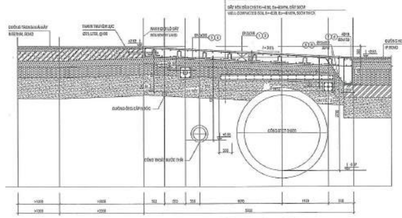
MẶT CẮT 2-2 (THI CÔNG MỚI) SECTION 2-2 (NEW CONSTRUCTION)
